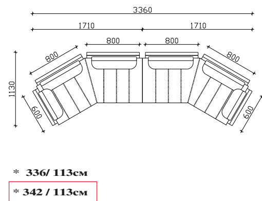
АГОЛ СО НАСЛОН 171x113cm x 2ком
